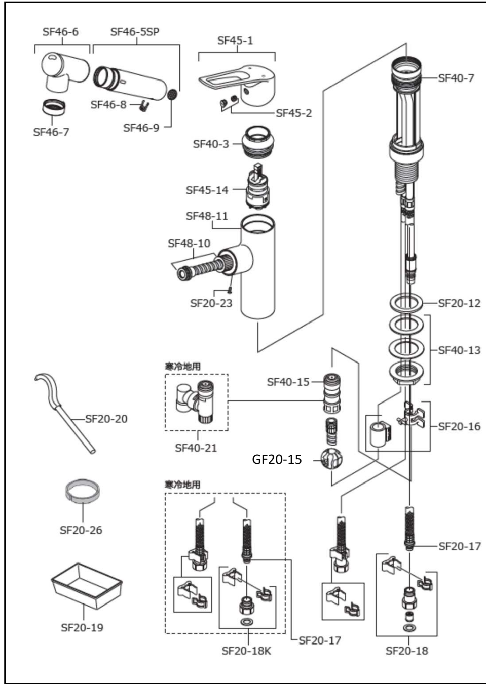
【部品構成図】
