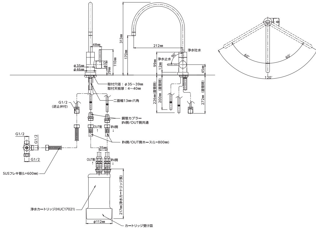
A113HU寸法図
